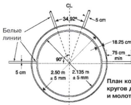
План круга для метания молота
